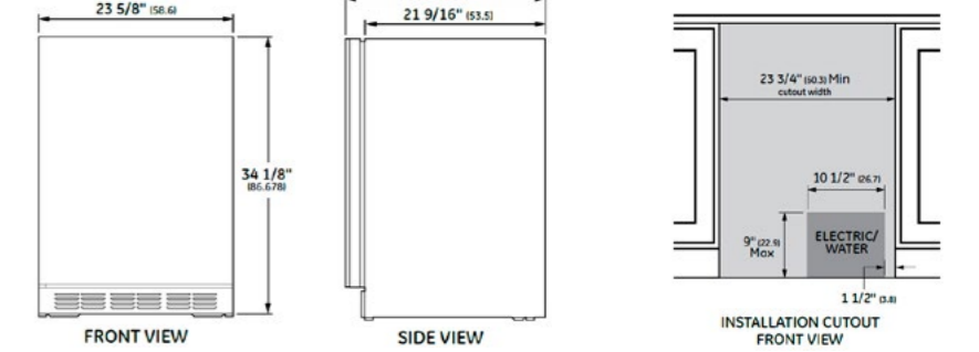
CAJÓN REFRIGERANTE: ZIDI240HII
